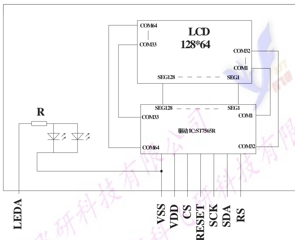
图 2：COG12864C1017图像点阵型液晶模块的电路框图
