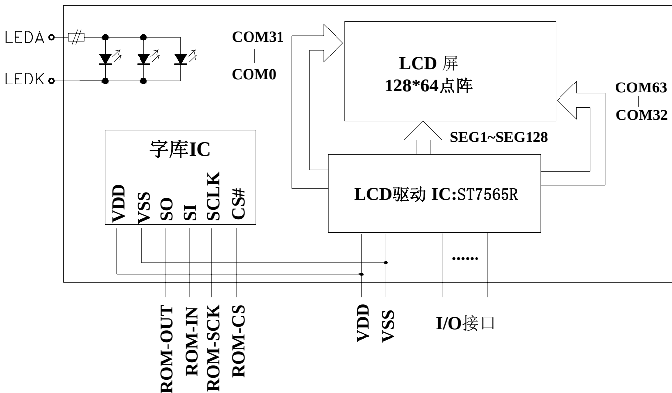
图 2: 电路框图
