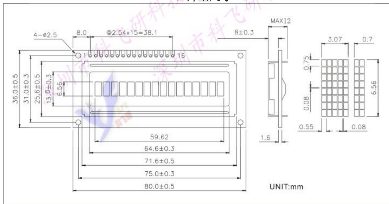
1X16 尺寸图
