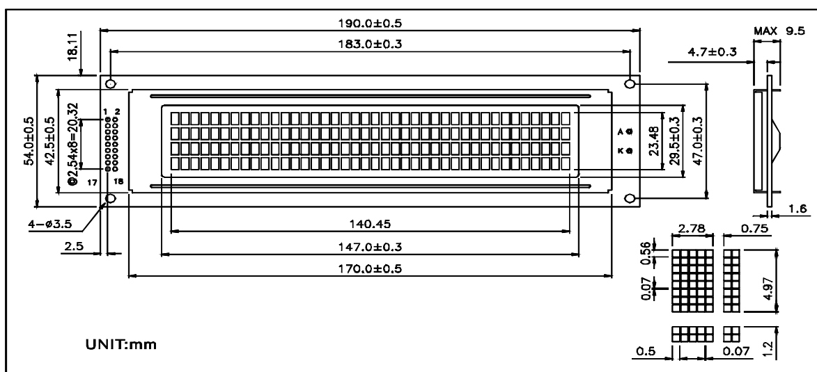
4X40 尺寸图
