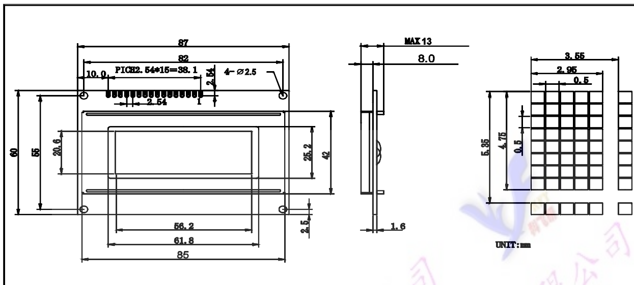
4X16 尺寸图
