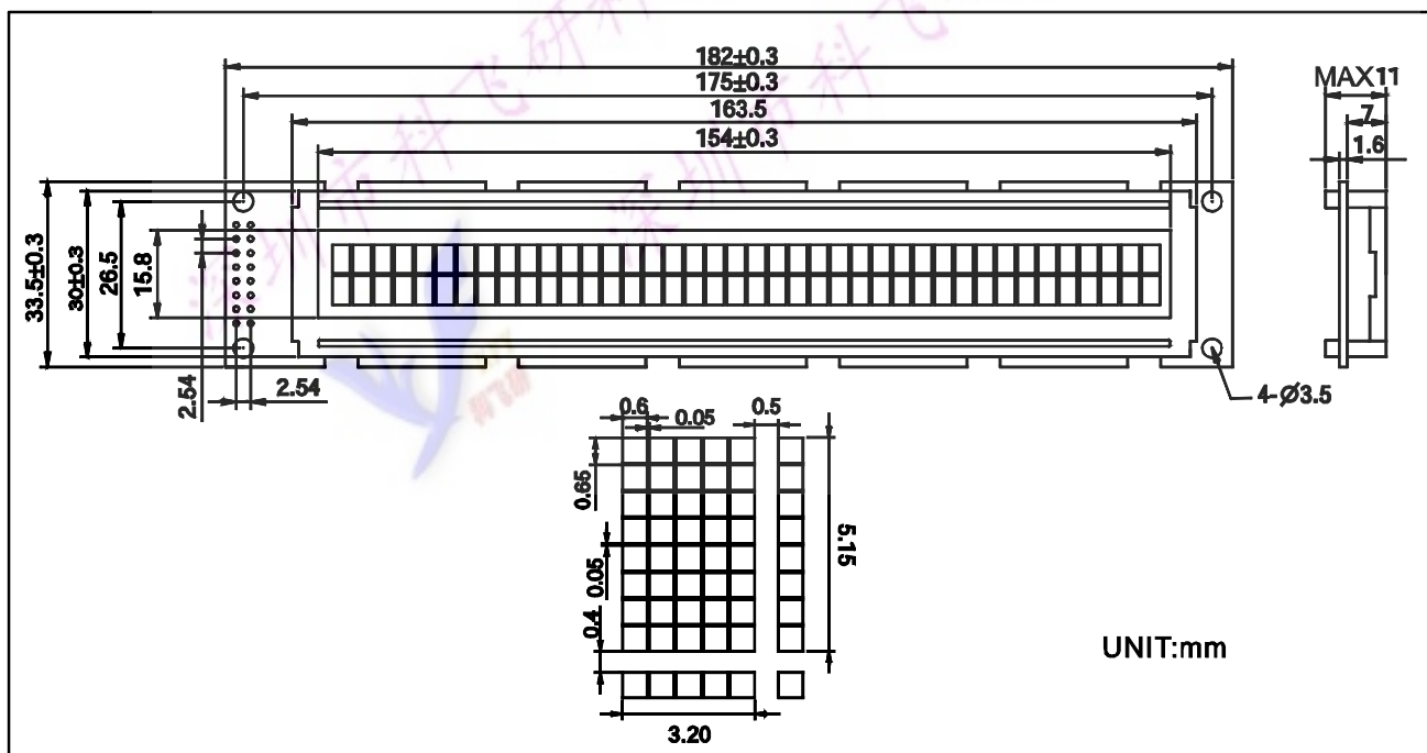
2X40 尺寸图
