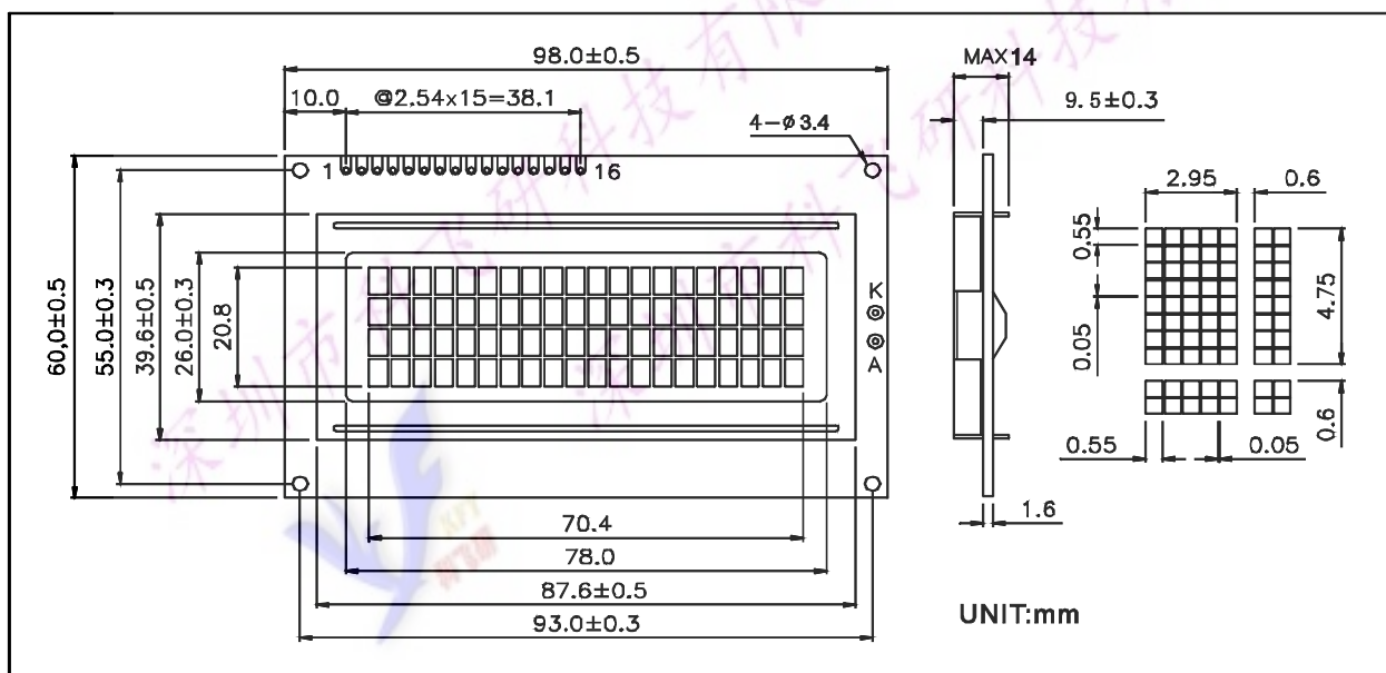
4X20 尺寸图
