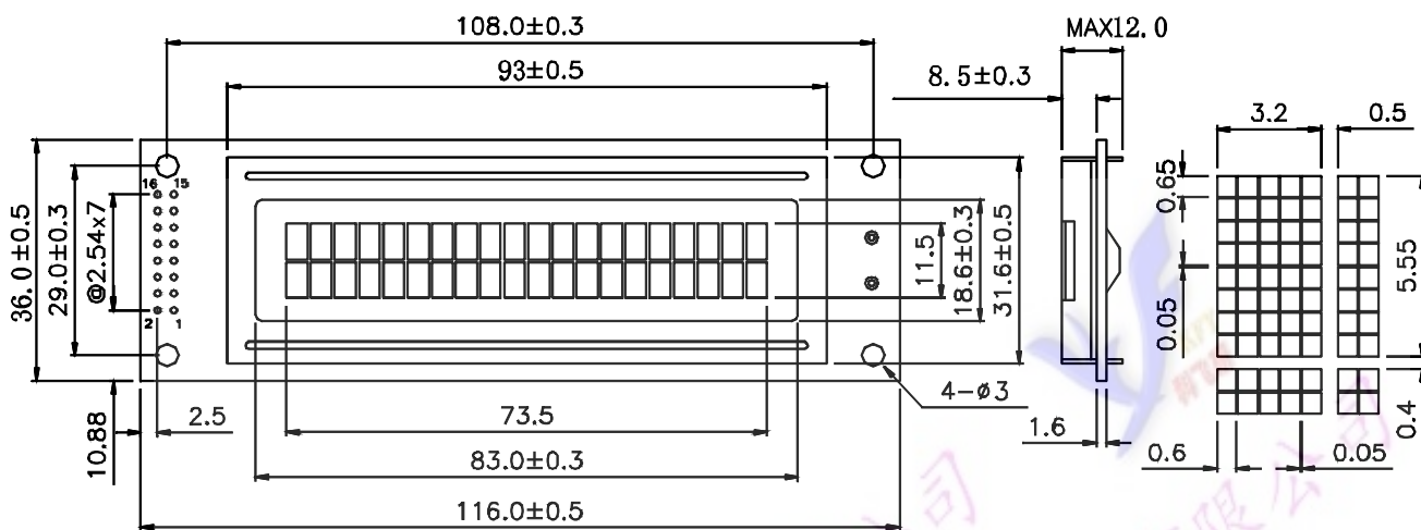
2X20 尺寸图
