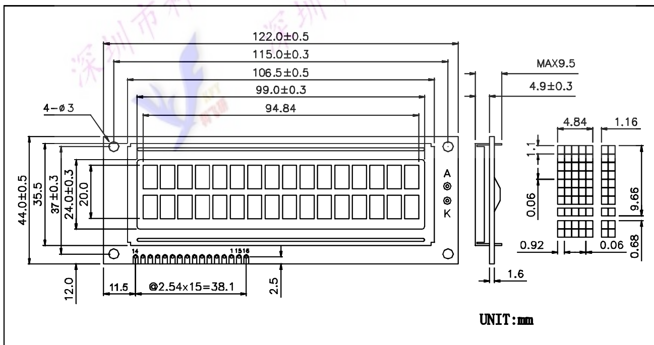
2X16B 尺寸图
